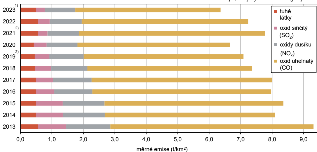
Měrné emise hlavních znečišťujících látek do ovzduší (REZZO 1–4) v Plzeňském kraji
