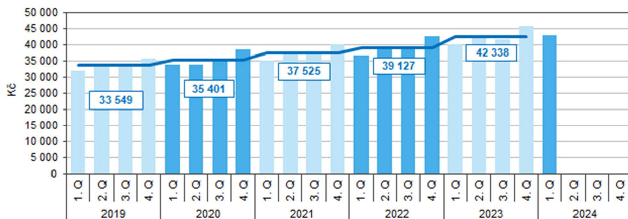
Graf 2 Vývoj průměrné měsíční mzdy v Jihomoravském kraji podle čtvrtletí
