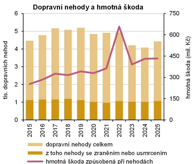
Graf 2.35 Dopravní nehody v Královéhradeckém kraji
