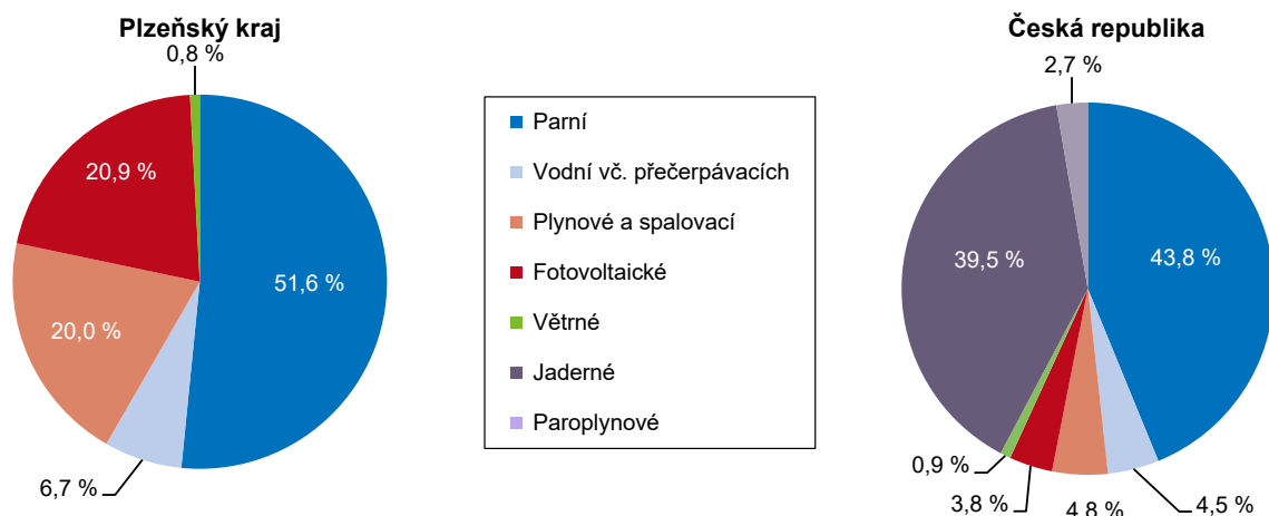
Graf 3.15 Výroba elektřiny brutto 1) podle technologie elektráren v roce 2023
