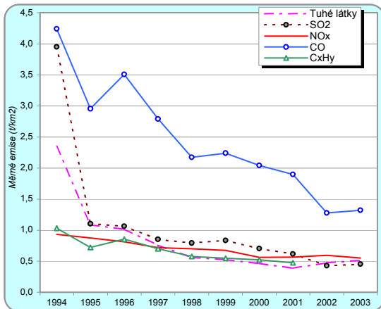
Vývoj měrných emisí hlavních znečišťujících látek
