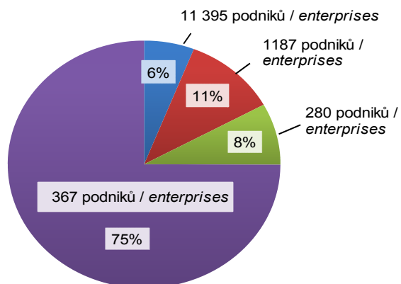
Graf 12 Počet podniků a jejich podíl na produkci podnikových odpadů podle množství vyprodukovaných odpadů v roce 2018 The number of enterprises and their share in waste generation according to the amount of produced waste in 2018
