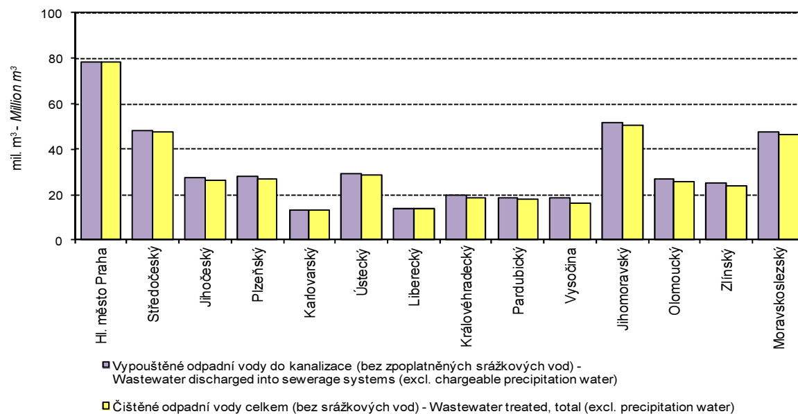
Množství vypouštěných a čištěných odpadních vod v jednotlivých krajích v roce 2016 Amount of wastewater discharged and treated: by region, 2016
