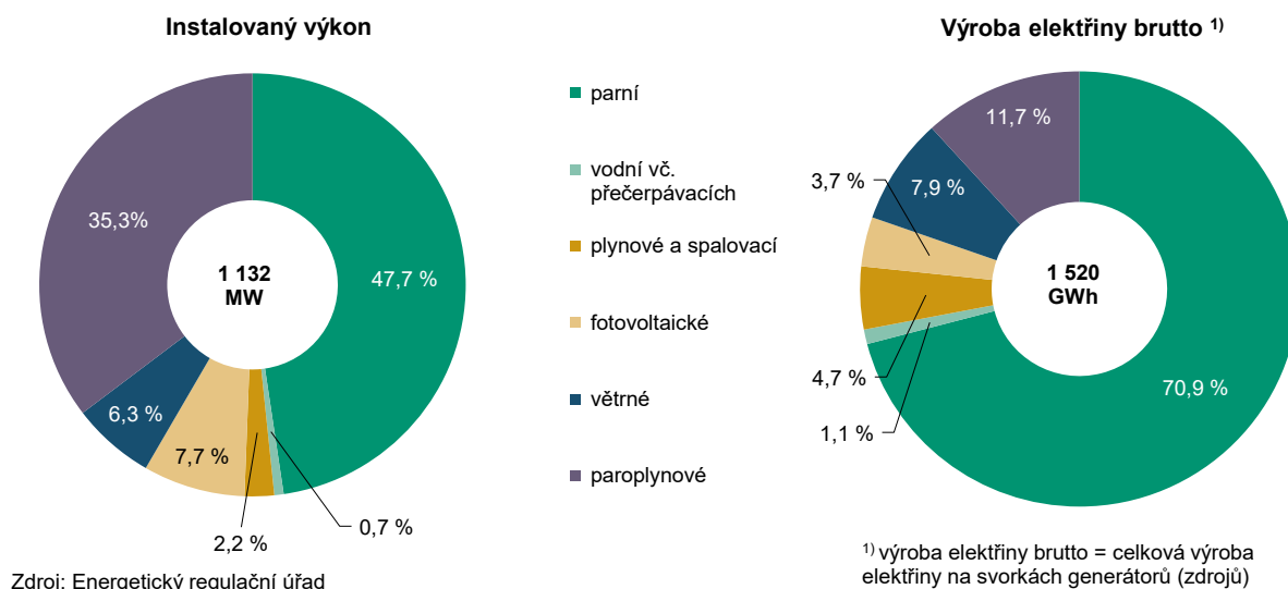
Graf 3. 24 Instalovaný výkon a výroba elektřiny podle technologie elektráren v Karlovarském kraji v roce 2025
