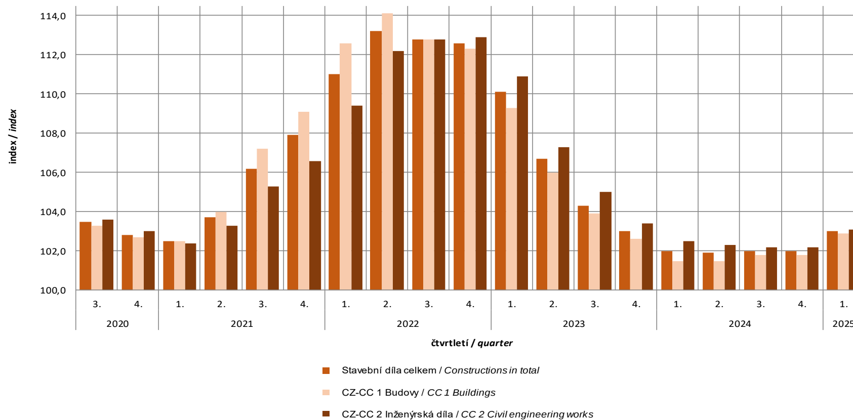
Graf 1: Indexy cen stavebních děl / Price indices of Constructions meziroční změny / year-on-year changes
