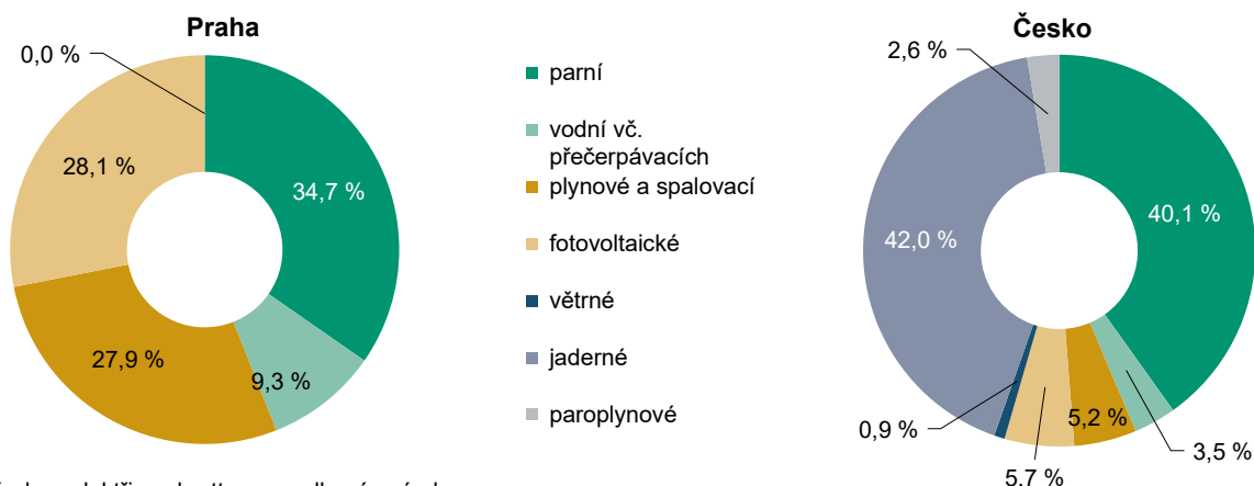
Graf 3.14 Výroba elektřiny brutto 1) podle technologie elektráren v roce 2025
