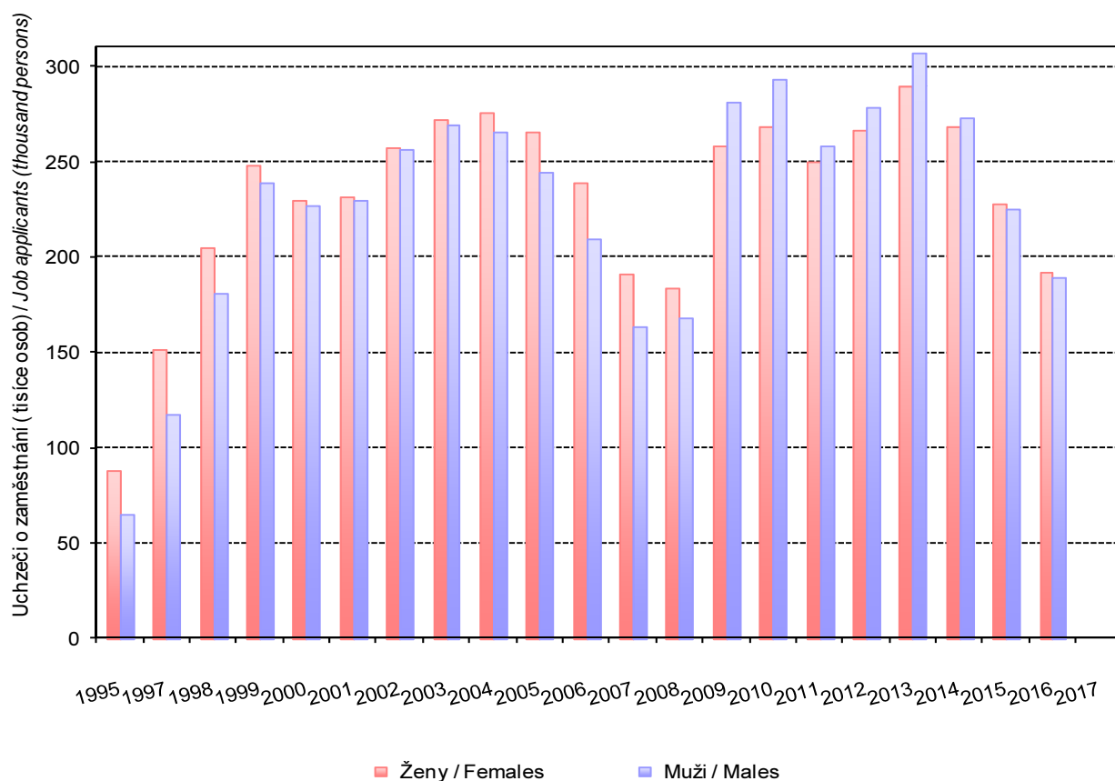
Graf 4-2 Neumístění uchazeči o zaměstnání k 31. 12. Job applicants kept in the labour office register as at 31 December
