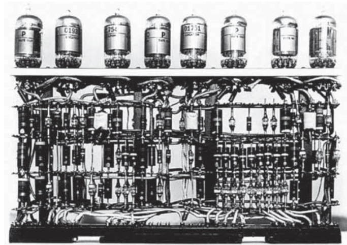
Součást počítače ABC s 8 elektronkami
