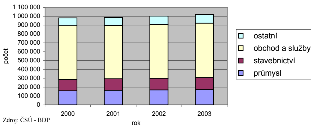
Graf č. 7: Struktura aktivních podniků
