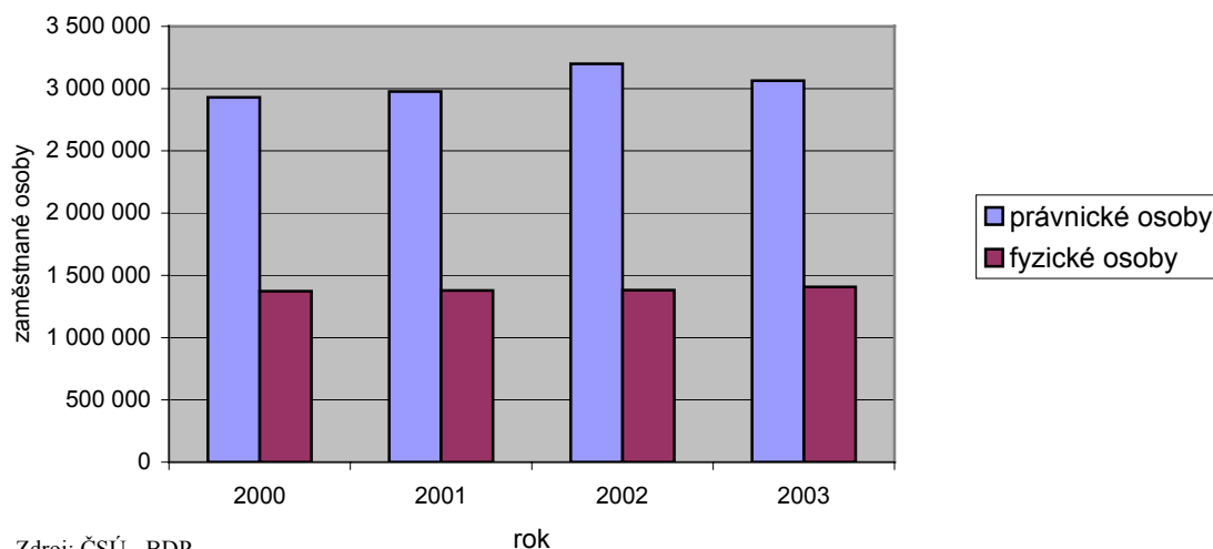
Graf č. 8: Zaměstnané osoby v aktivních podnicích
