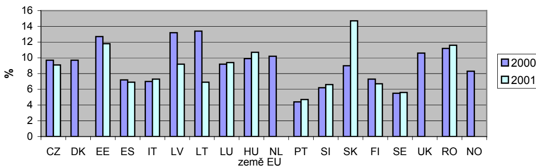
Graf č. 11: Podíly zániků v zemích EU
