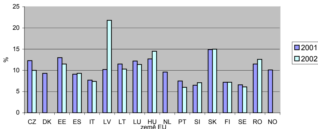
Graf č. 9 : Podíl vzniků v zemích EU
