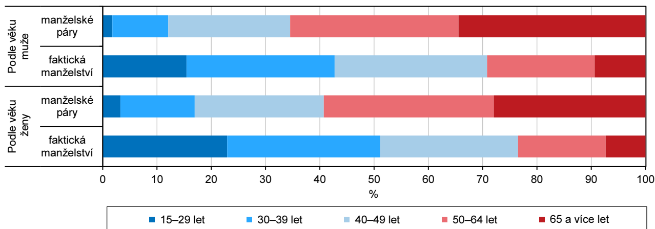
Graf 6.2.5 Manželské páry a faktická manželství podle věku partnerů (hospodařící domácnosti tvořené 1 rodinou)
